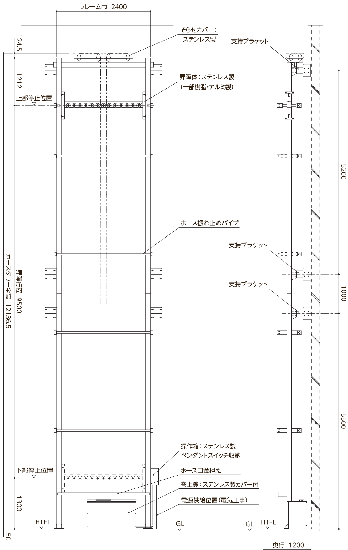
正面図
